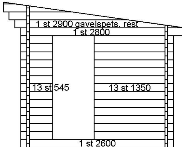
MELLANVÄGG MED BASTUDÖRR
