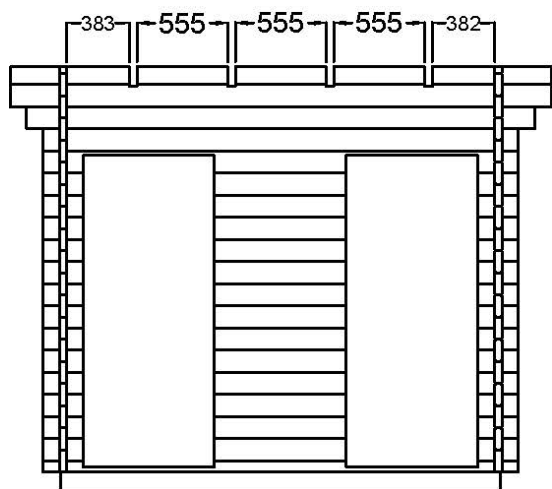
Framsida 1
