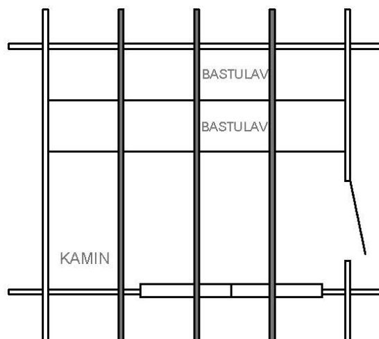
Vy uppifrån
