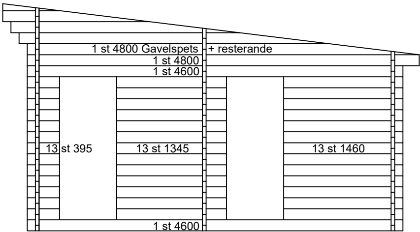
Mellanvägg
