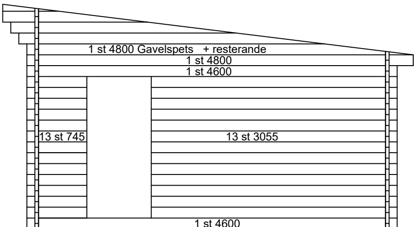
Gavelvägg ytterdörr
