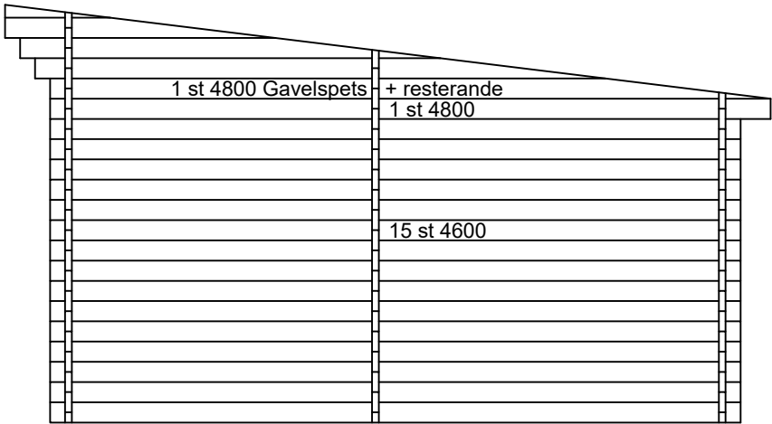
Gavelvägg bastu
