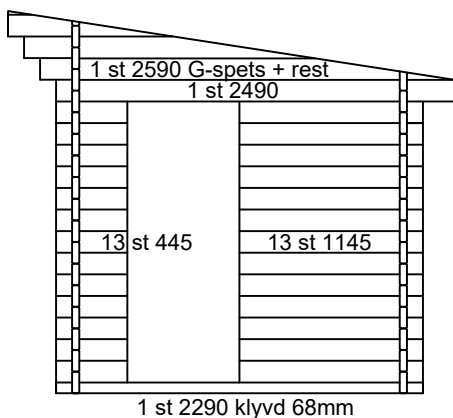
Gavelvägg omkläd.
