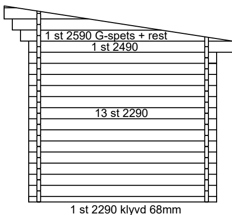
Gavelvägg bastudel
