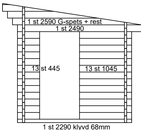
Gavelvägg omkläd.
