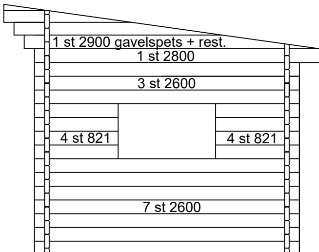
Gavelvägg omkläd.
