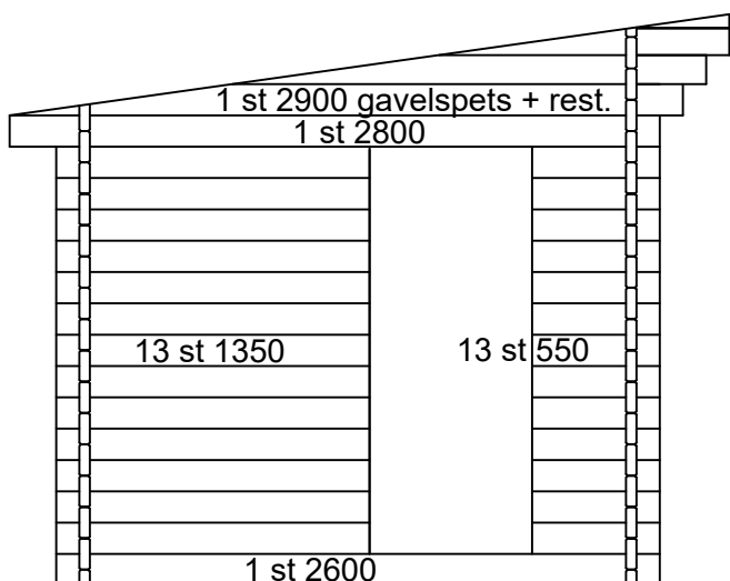
Mellanvägg
