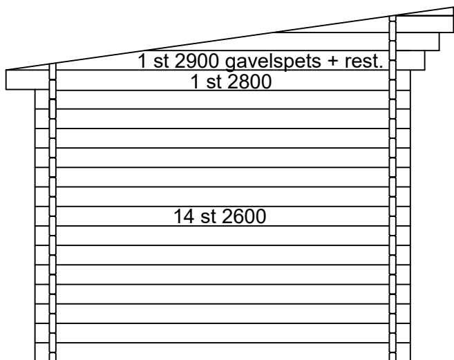
Gavelvägg bastudel
