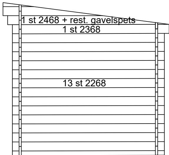
1 st 2268 som är klyvd 68mm
