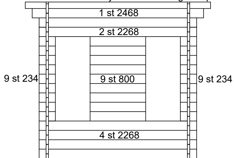
1 st 2668 som måste klyvas i nivå med gavelspets
